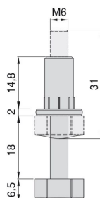
CROQUIS
