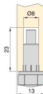
MONTAJE
