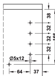
Esquema de taladro armario
