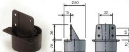
Base de fijación con escuadra
