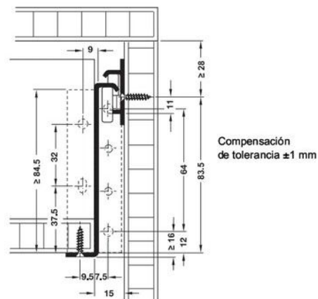
Montaje
